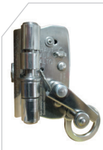
Freno de acero inoxidable con traba para cuerda de 11 a 13 mm.
