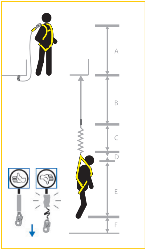
Ejemplo del cálculo de altura libre necesaria para detener una caída de factor 2
