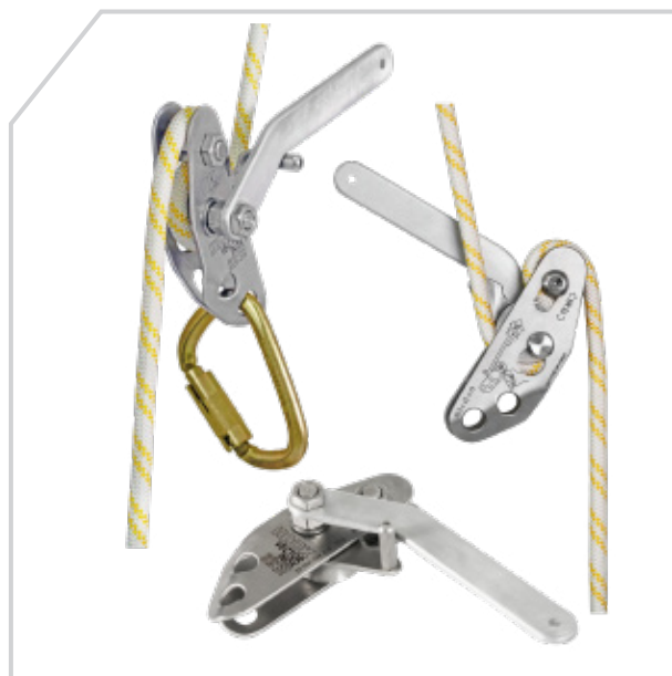
Descendedor autobloqueante Tipo C - Vector H1 de acero inoxidable
